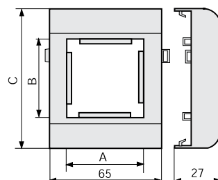
Рамка-суппорт PDA-45N для коробов шириной 80 мм
