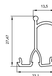
Разделитель для короба SEP-N40
